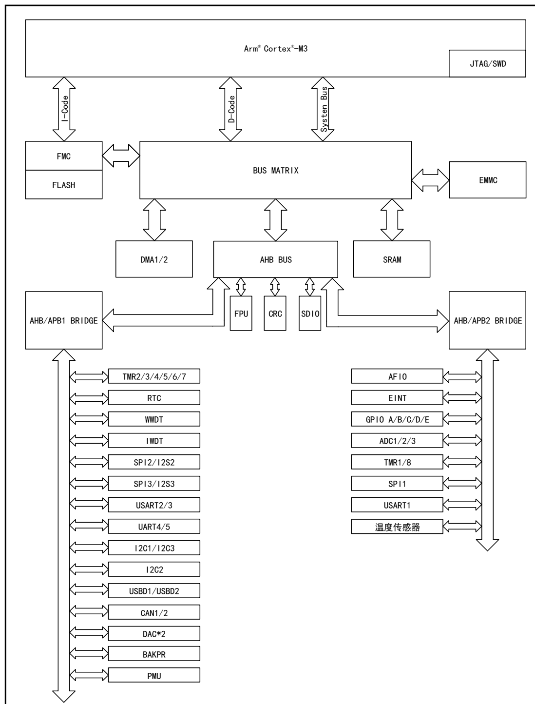
图 3 APM32A103xET7 系统框图
