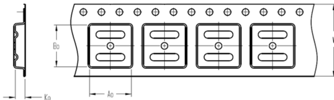
图 21 带状包装规格图
