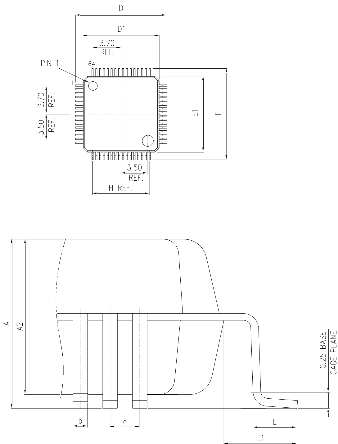
图 18 LQFP64 封装图
