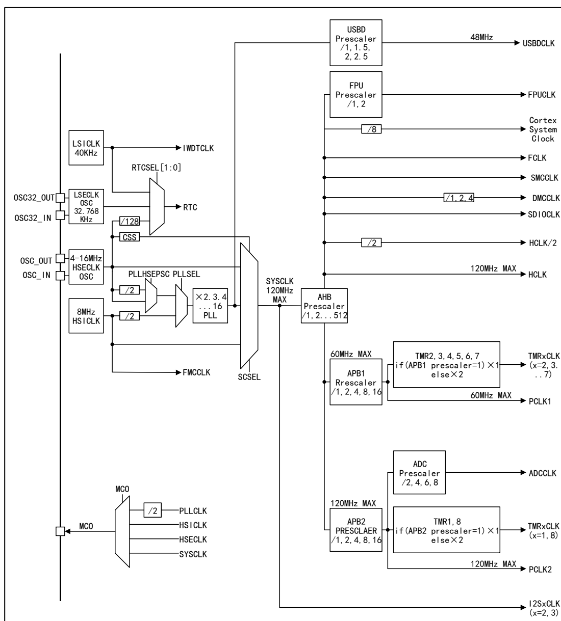
图 5 APM32A103xET7 时钟树
