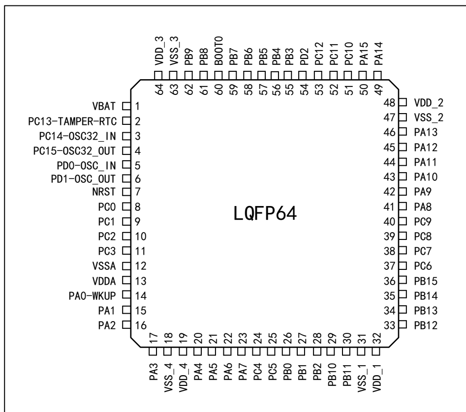
图 2 APM32A103xET7 系列 LQFP64 引脚分布图
