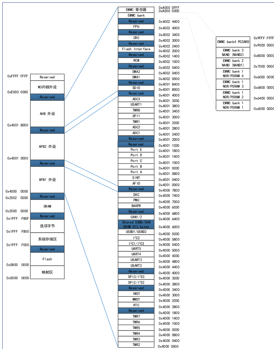
图 4 APM32A103xET7 系列地址映射图
