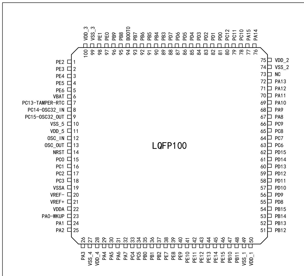
图 1 APM32A103xET7 系列 LQFP100 引脚分布图
