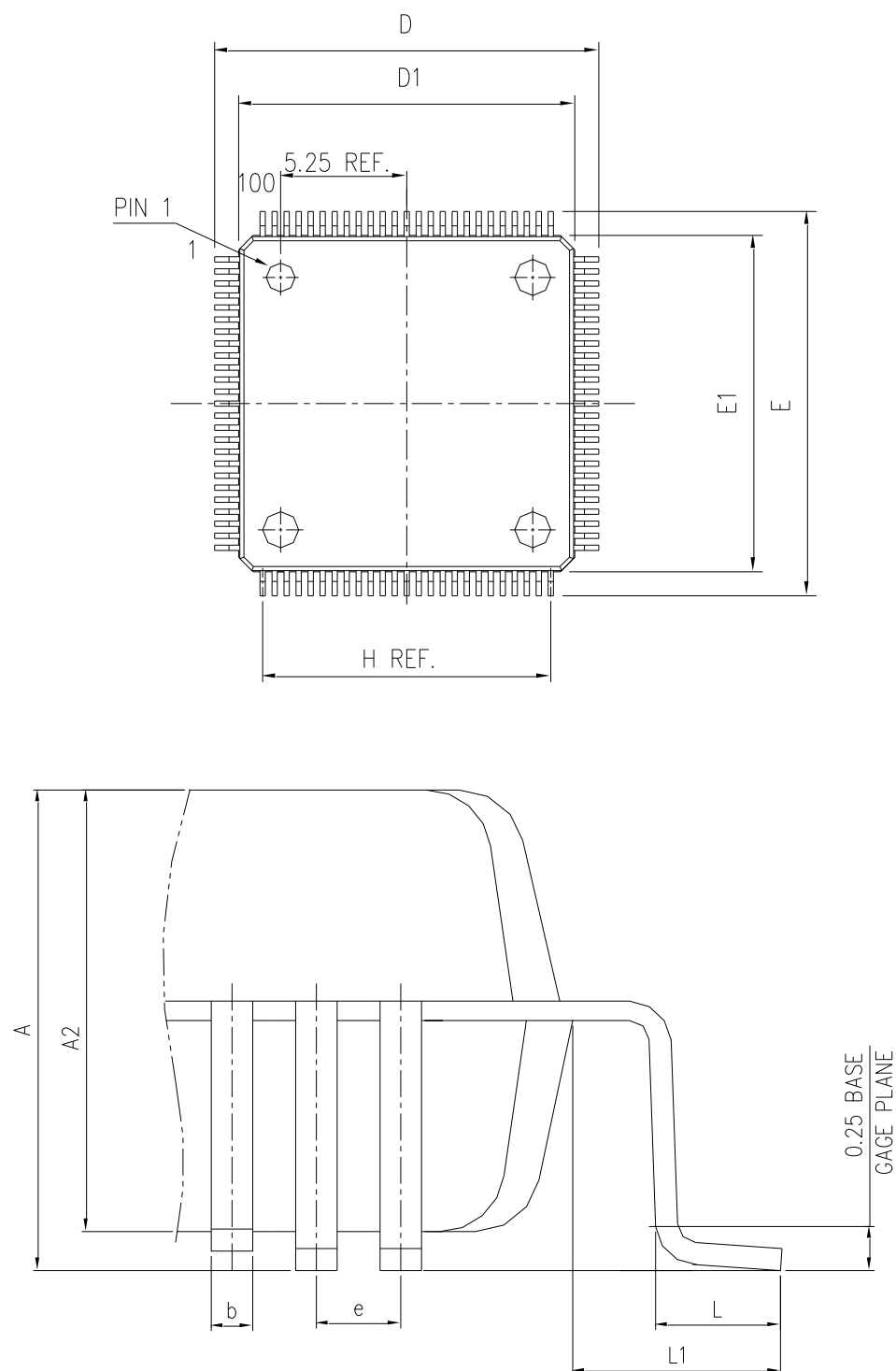
图 15 LQFP100 封装图
