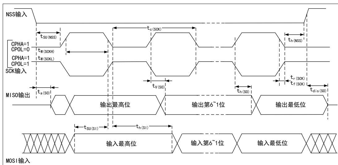
图 13 SPI 时序图—从模式和 CPHA=1
